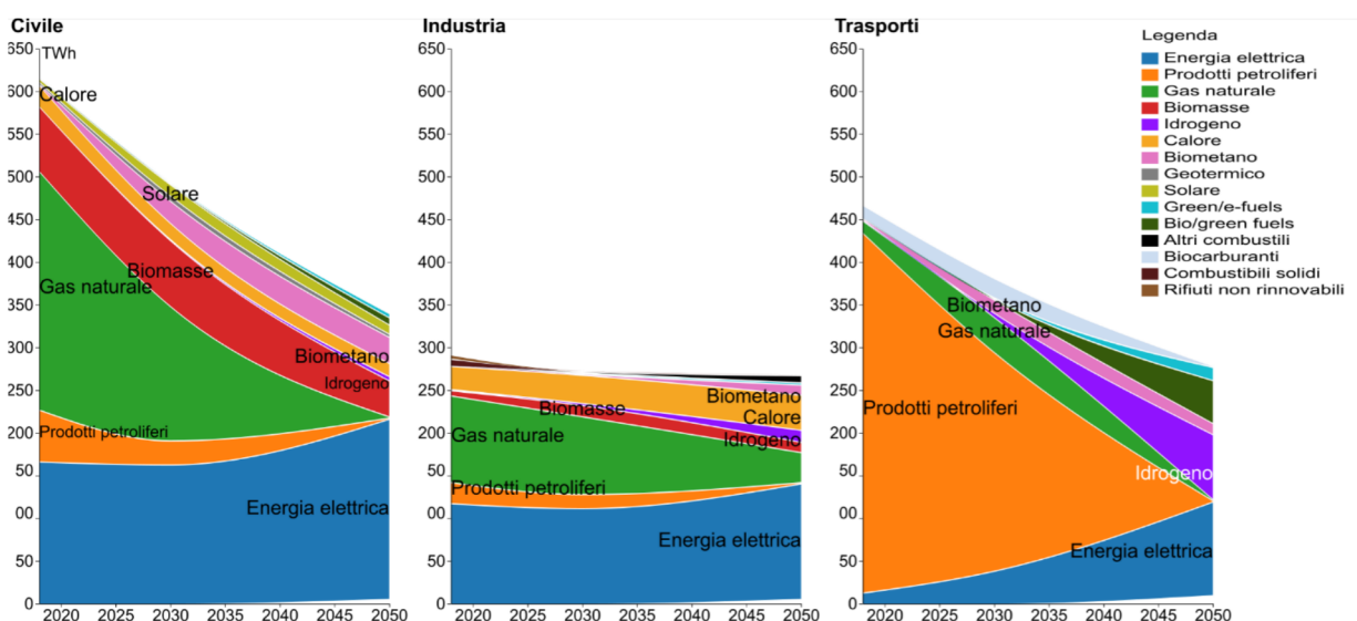
Figura 9. Evoluzione del mix energetico per macro-settori 2020 – 2050. Elaborazioni MITE su dati RSE. 60
