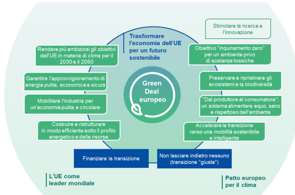
Figura 3. Schema del Green Deal europeo.
