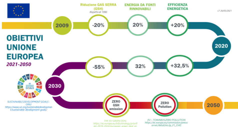
Figura 4. Roadmap obiettivi europei di decarbonizzazione al 2030 e 2050.
