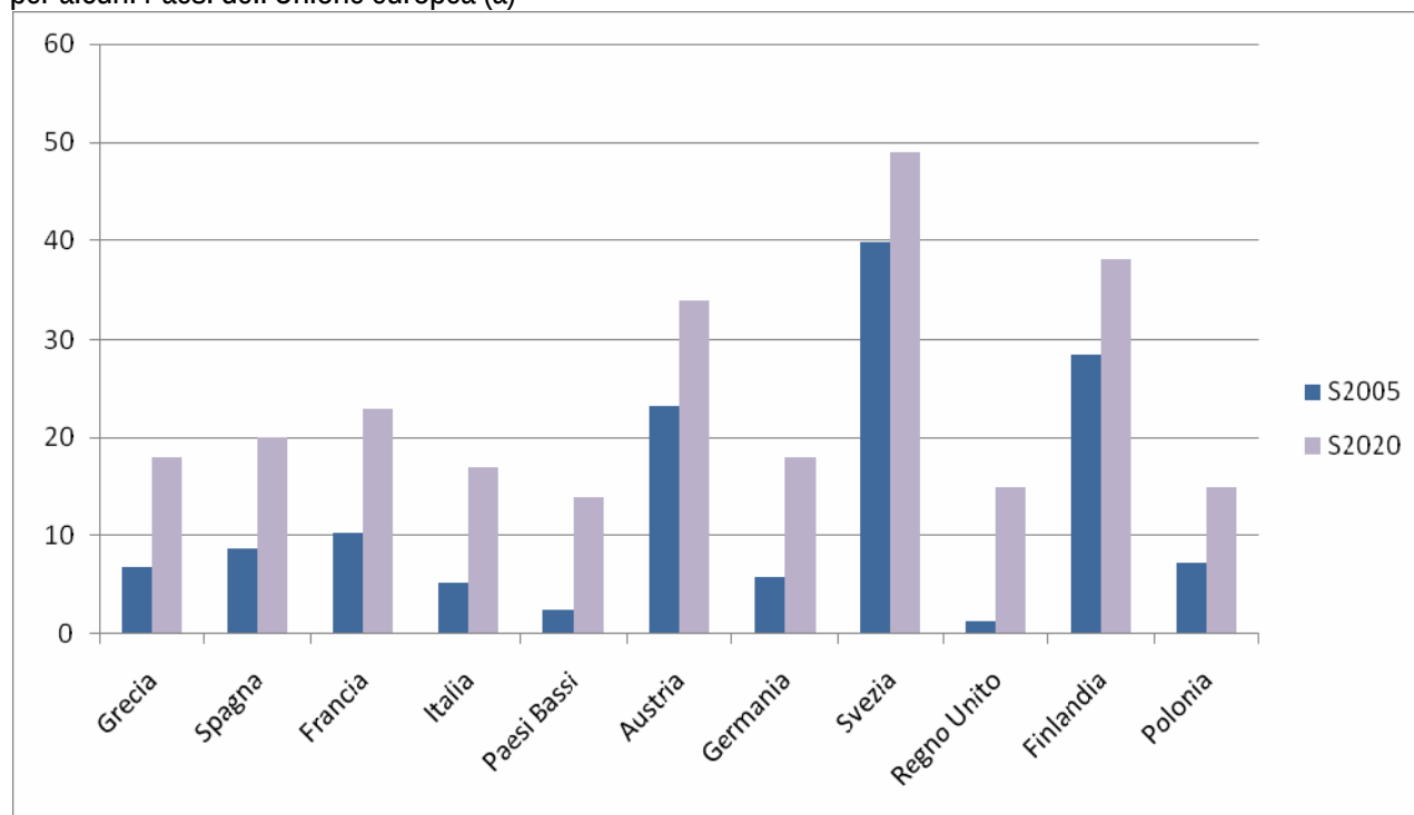
Figura 2 - Obiettivi nazionali per la quota di energia da fonti rinnovabili sul consumo finale di energia nel 2020 per alcuni Paesi dell'Unione europea (a)
