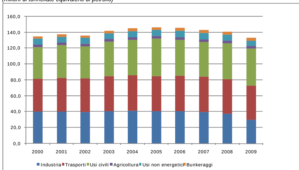
Figura 5 – Usi finali di energia nei settori d'uso - Anni 2000 – 2009 (a) (milioni di tonnellate equivalenti di petrolio)
